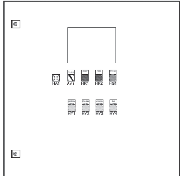
Рис. 9 Прибор управления пожарной Control MX
