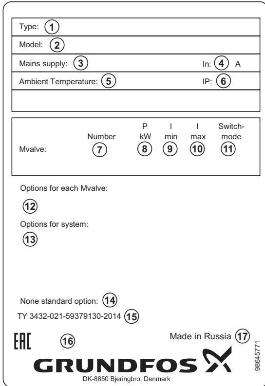
Рис. 2 Фирменная табличка Control VLV
