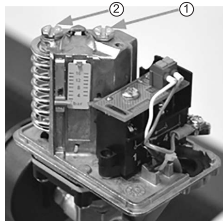
Рис. 5 Настройка реле давления FRG
