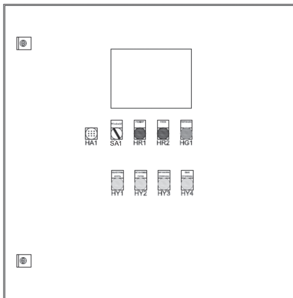
Նկար 9 Control MX կառավարման հրշեջ սարք
