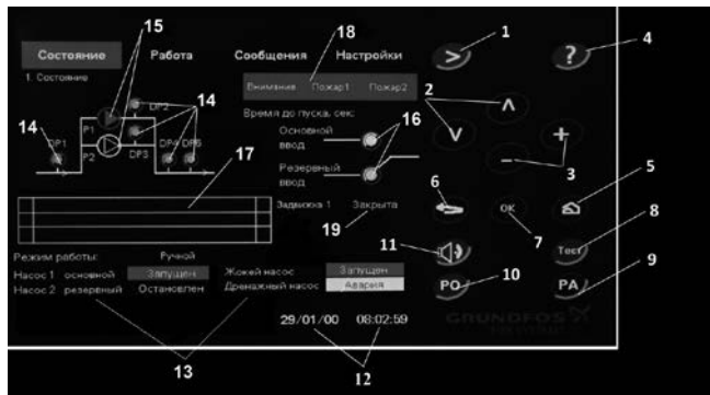
Рис. 13 Меню «Состояние»
