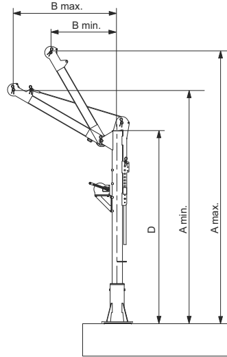
Рис. 12 Размеры крана
