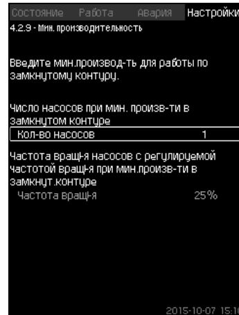
Рис. 61 Мин. производительность
