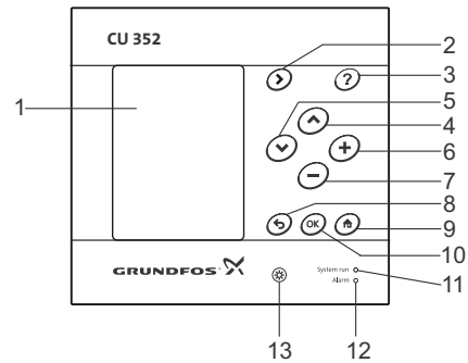
Рис. 4 Панель управления
