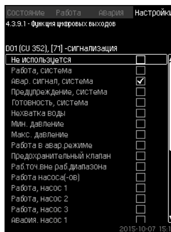
Рис. 78 Функция цифровых выходов
