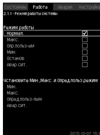
Рис. 18 Режим работы системы
