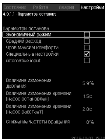
Рис. 68 Специальные настройки
