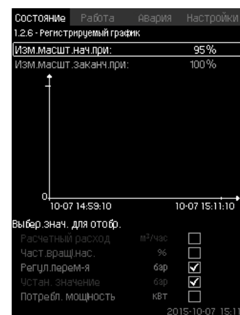
Рис. 14 Регистрируемый график
