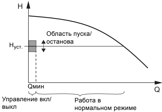
Рис. 65 Область пуска/останова
