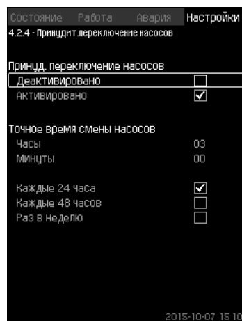
Рис. 56 Принудит.переключение насосов
