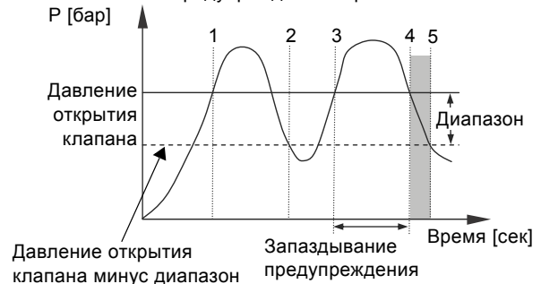
Рис. 105 Сброс давления
