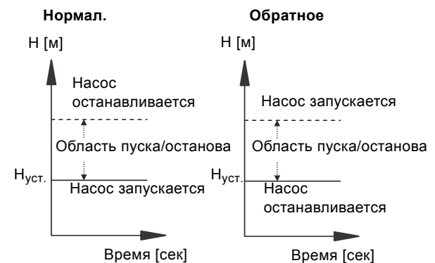
Рис. 50 Нормальное и обратное управление
