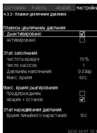
Рис. 69 Плавное увеличение давления
