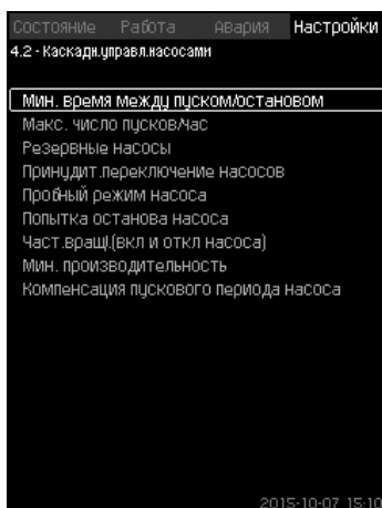
Рис. 52 Каскадн.управл.насосами
