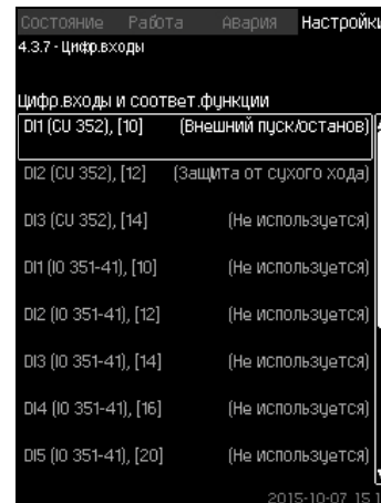
Рис. 72 Цифр.входы
