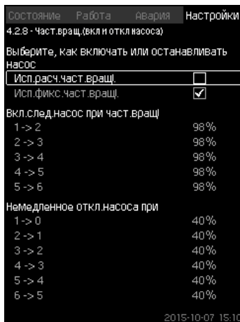
Рис. 60 Исп.фикс.част.вращ.
