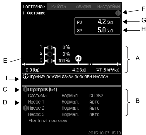
Рис. 6 Состояние
