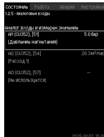
Рис. 13 Аналоговые входы
