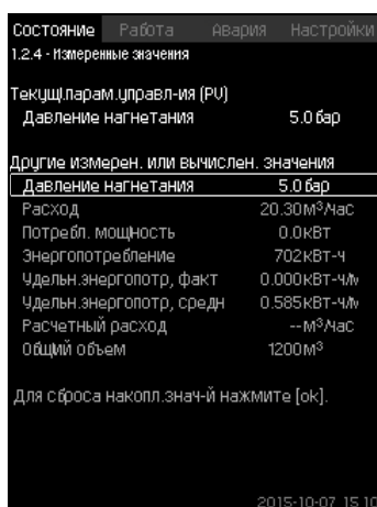
Рис. 12 Измеренные значения
