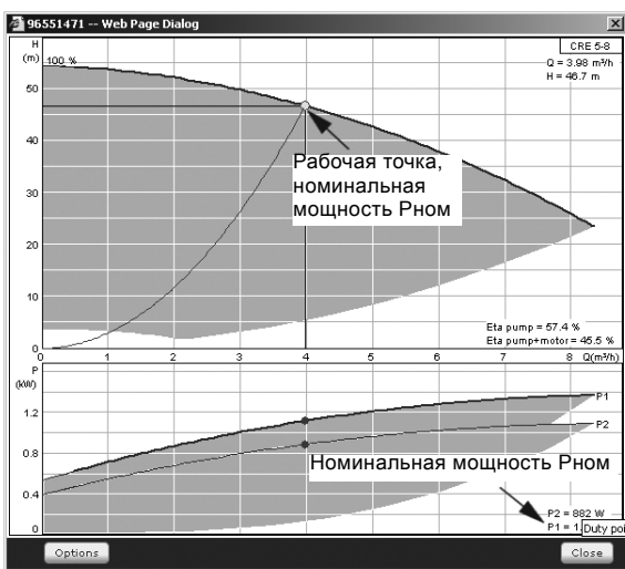
Рис. 89 Показание номинальной мощности Rном (WebCAPS)
