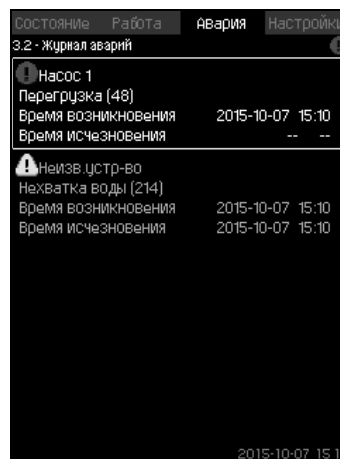
Рис. 34 Журнал аварий
