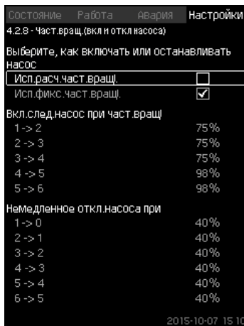
Рис. 59 Исп.расч.част.вращ.
