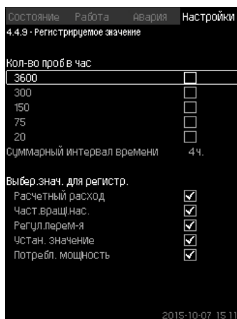
Рис. 106 Регистрируемое значение
