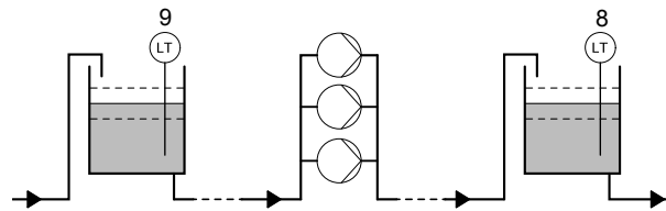
Рис. 127 Контроль уровня
