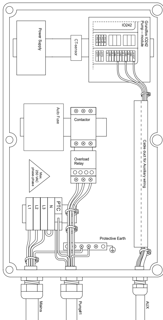
Трёхфазные подключения для одного насоса без нейтрали, только для Норвегии
