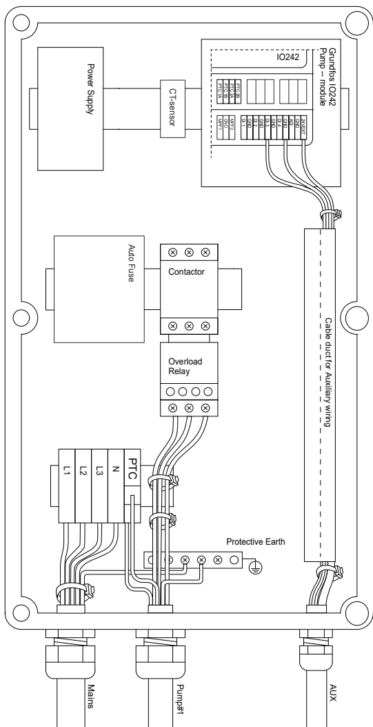
Трёхфазные подключения для одного насоса
