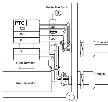
Рекомендованная проводка PTC
